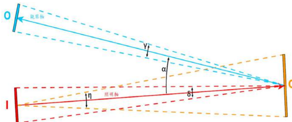
圖三：用於測量反光裝置之量測幾何形狀
