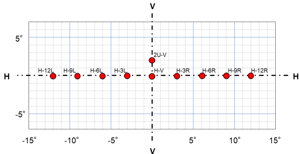
圖二：遠光光束測試點
