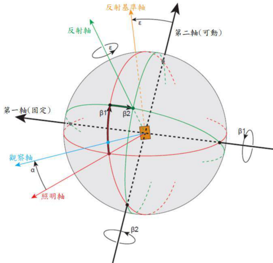
圖一：CIE 座標系統
