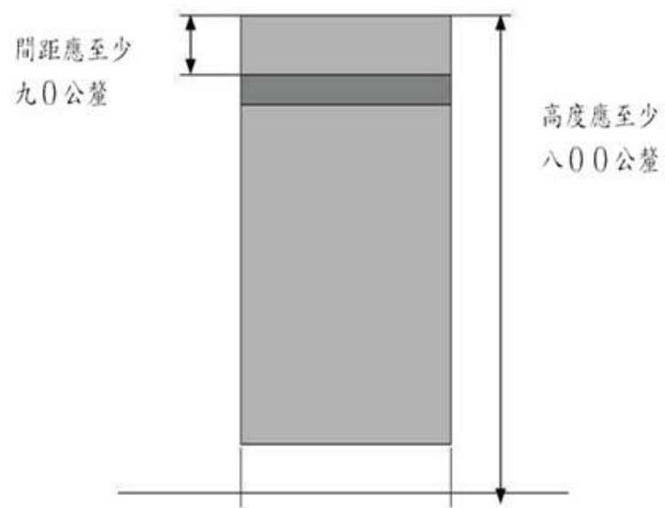
圖八：防護桿
