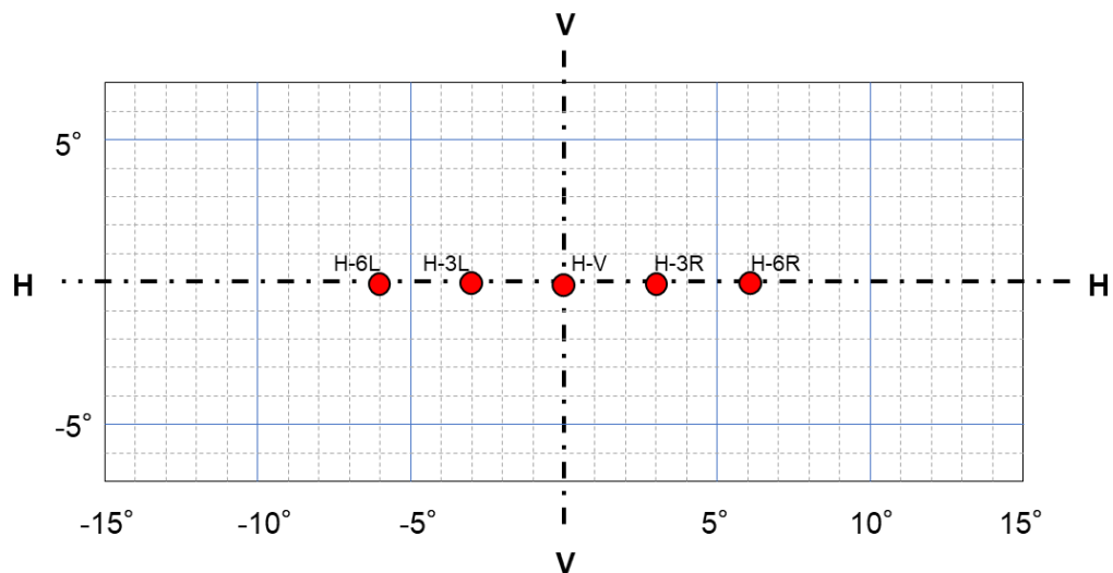
圖三：類型 BS 遠光光束-測試點位置
