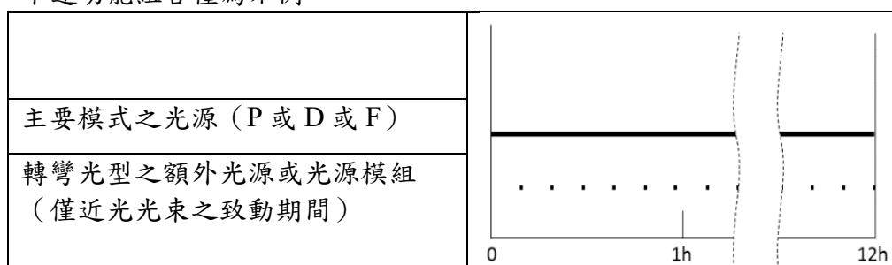
圖十七、配備單一照明功能及轉彎光型之頭燈範例
