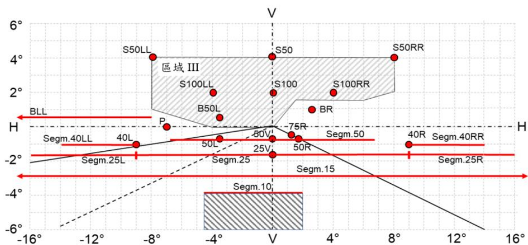
圖五：類型 C 及 V 近光光束
