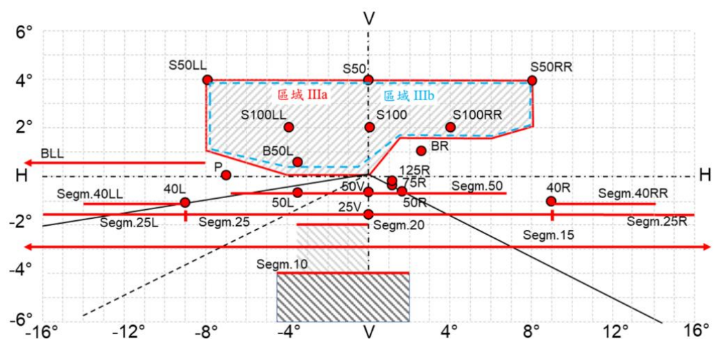
圖六：AFS 近光光束
