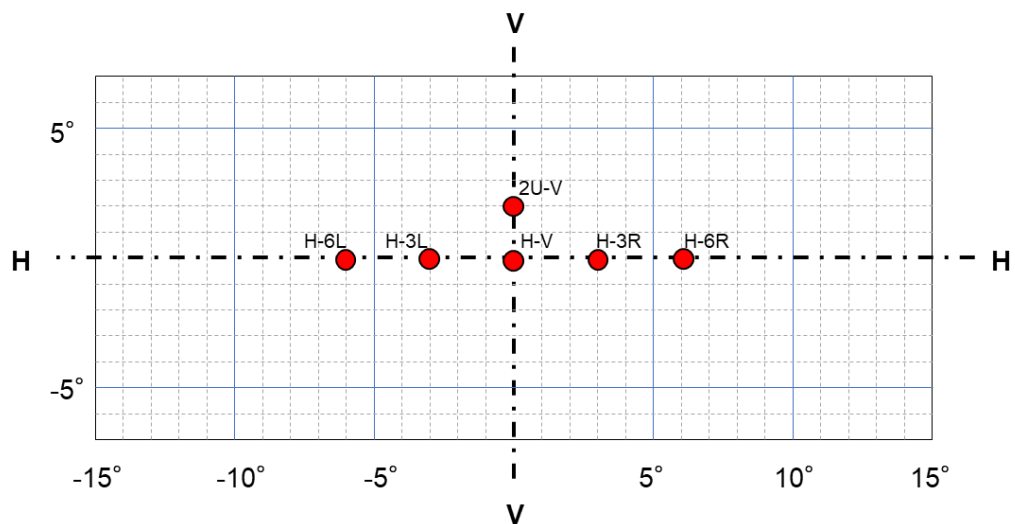
圖四：類型 CS 及 DS 次要遠光光束-測試點位置
