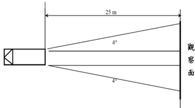
車輛後方反光標識可視性示意圖
