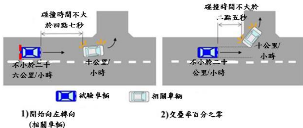
圖二、前行車輛右轉或左轉
