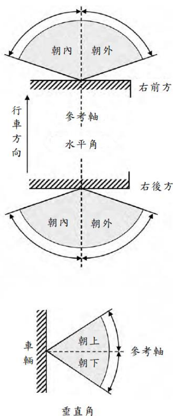
圖一：車寬燈、尾燈、輪廓邊界標識燈、煞車燈、前後方向燈、晝行燈及前後停車燈 光度分佈角度-水平與垂直
