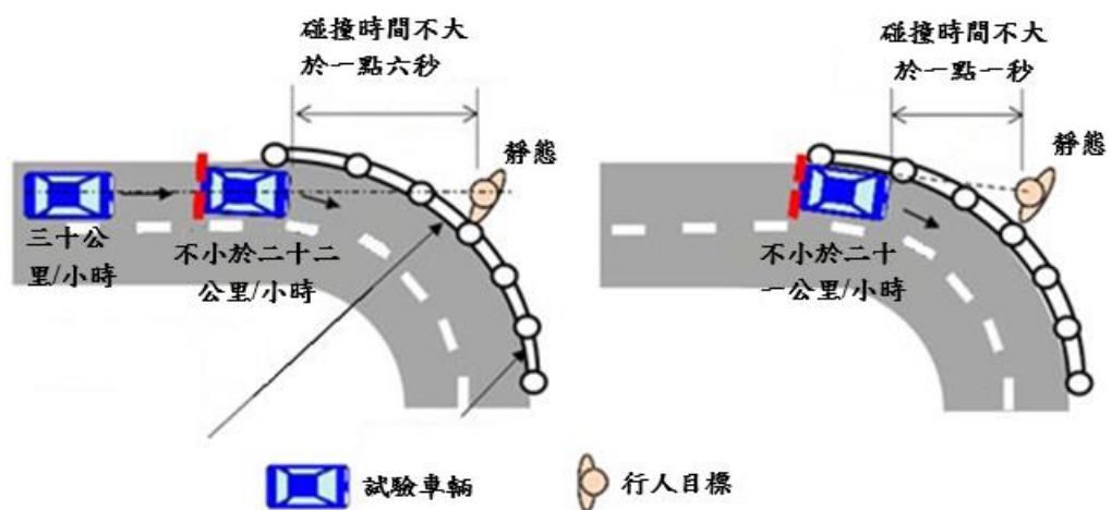
圖三、具備護欄之彎道及一靜態物體
