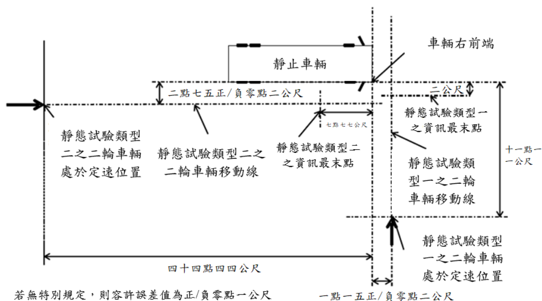
圖二 靜態試驗
