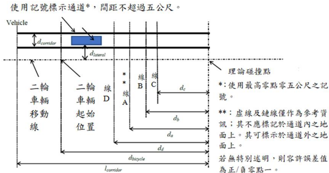
圖二 靜態試驗
